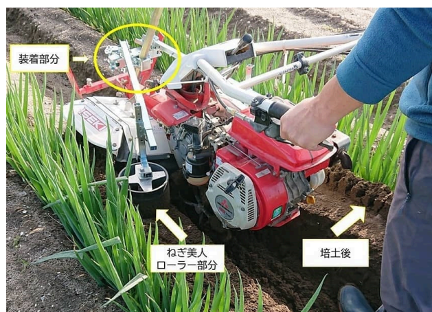
管理機取付後 土寄せ作業の様子
